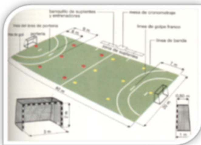
Dimensiones y medidas del terreno de juego
