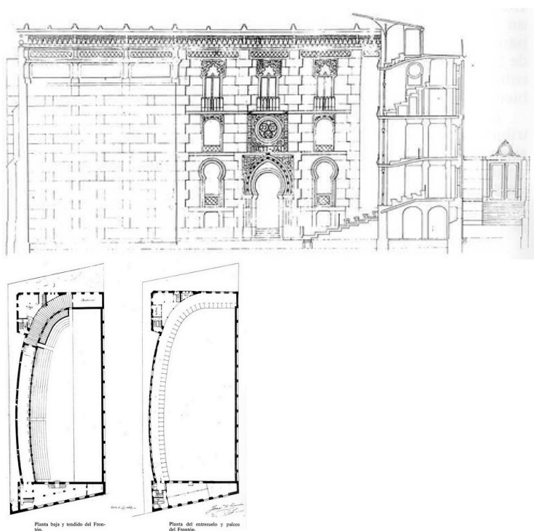
Plano de la fachada interior del frontón y sección de palcos Detalles Planos del Edificio
